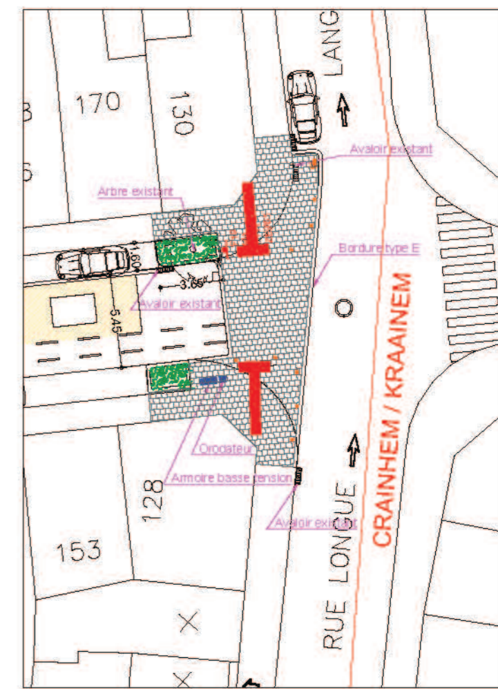
Effets de porte matérialisés par deux bacs à plantes carrefour Hinnisdael, zone franchissable + bacs à plantes Carrefour Bonheur
