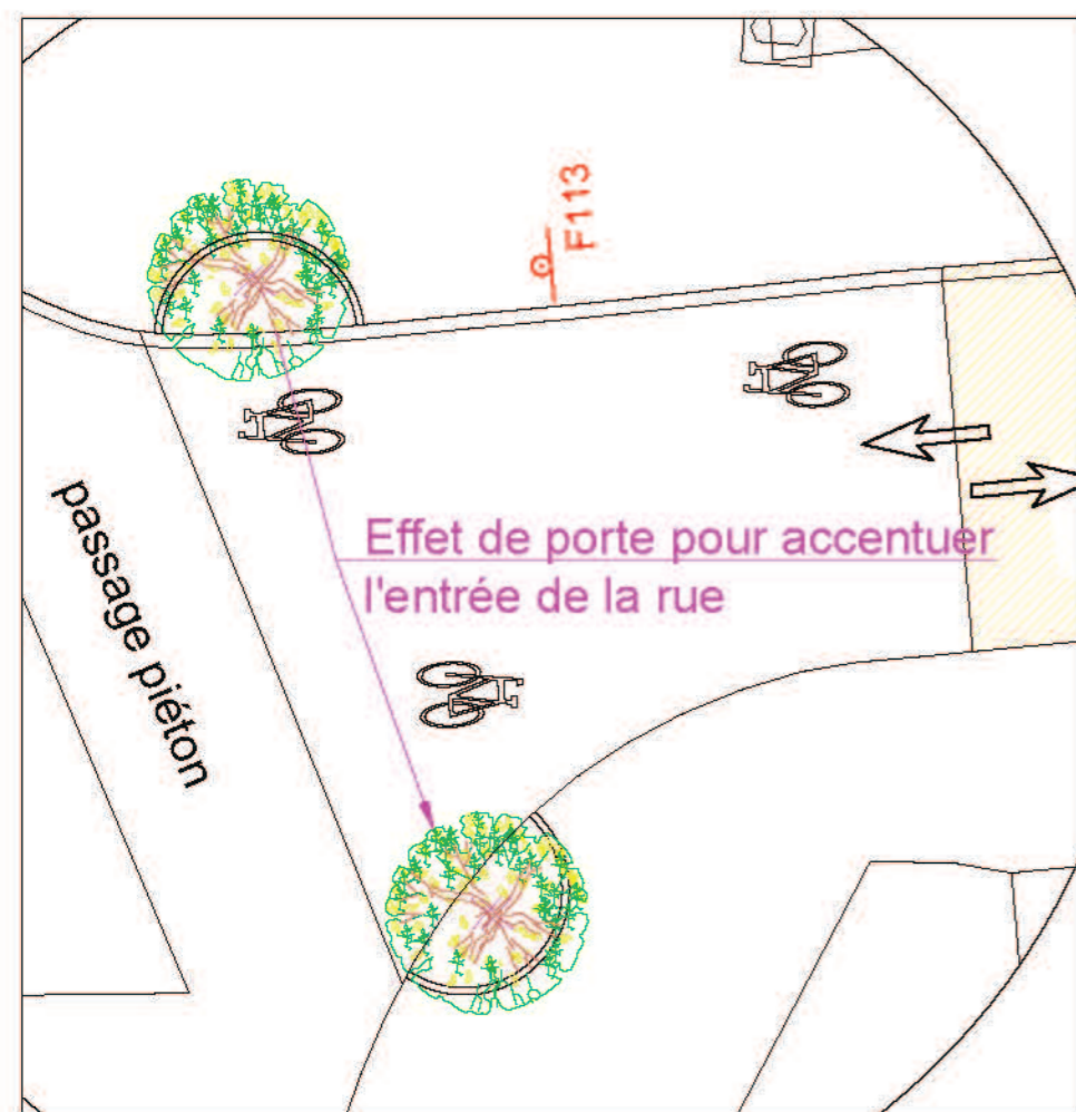
Effets de porte matérialisés par deux bacs à plantes carrefour Hinnisdael, zone franchissable + bacs à plantes Carrefour Bonheur
